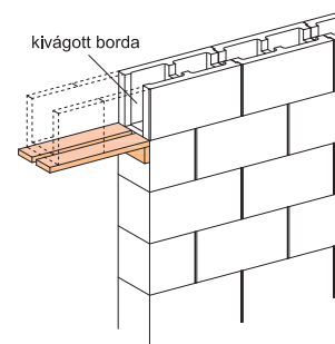
18. Kivágott elemborda nyílásáthidalásnál
