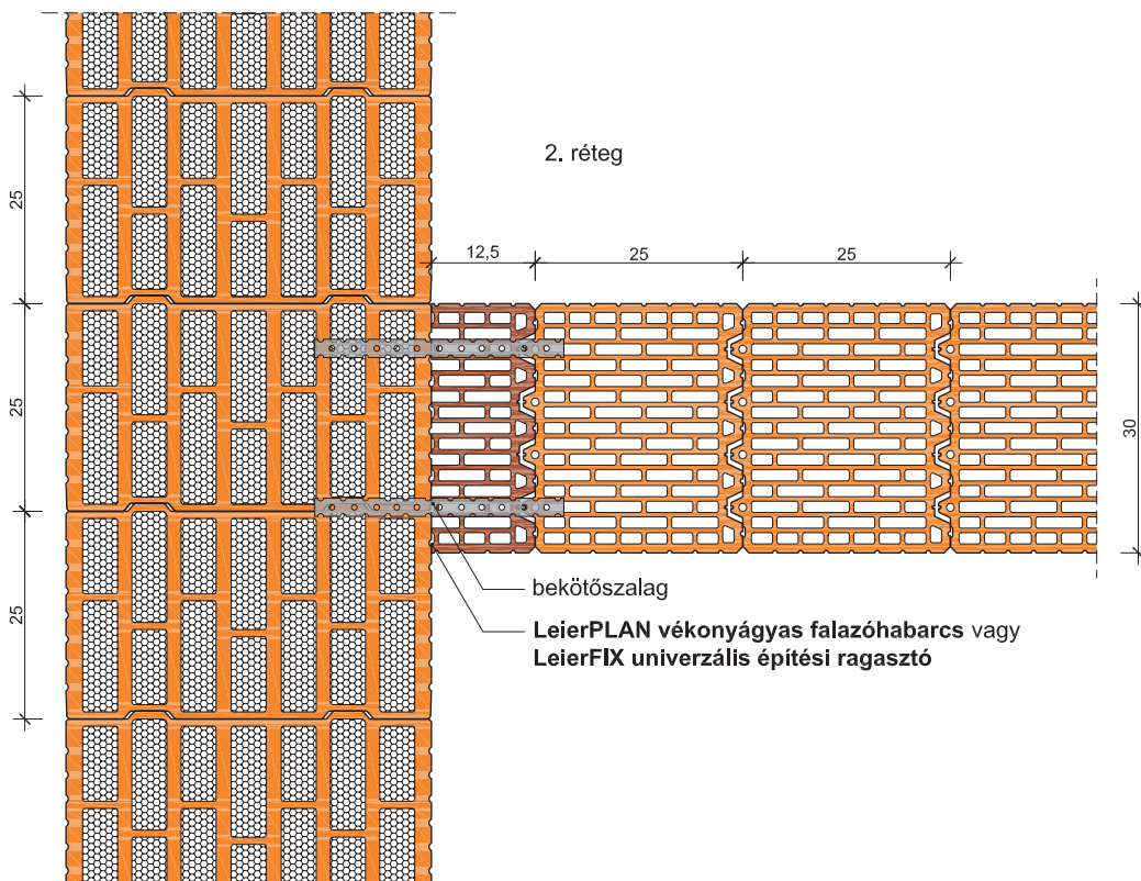
77. Falcsatlakozás: LeierPLAN 44 iSO + – LeierPLAN 30 N+F / LeierPLAN 44 iSO + – LeierPLAN 30 Pro LeierPLAN 44 Pro – LeierPLAN 30 N+F / LeierPLAN 44 Pro – LeierPLAN 30 Pro
