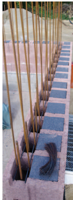
11. Durisol falszerkezet építése erősítő vasalással
