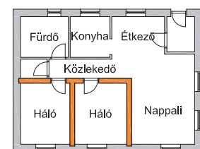
29. Nyugodt és zajos zónát elválasztó falak
