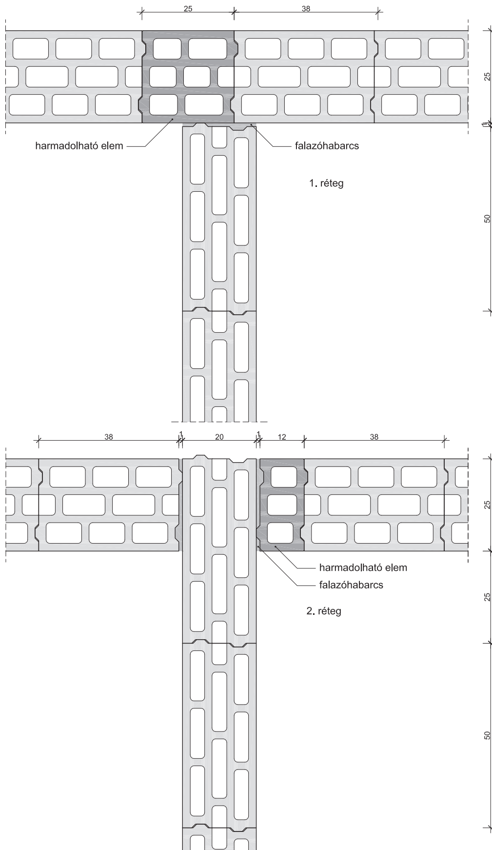
20. Falcsatlakozás: Leier beton főfalelem FF 25 – Leier beton főfalelem FF 20
