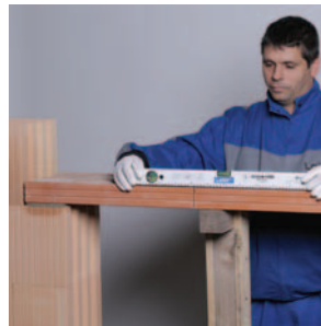
49. Vízszintes helyzet ellenőrzése
