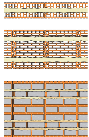
12. LeierFIX univerzális építési ragasztó felhordása különböző falazóelemekre
